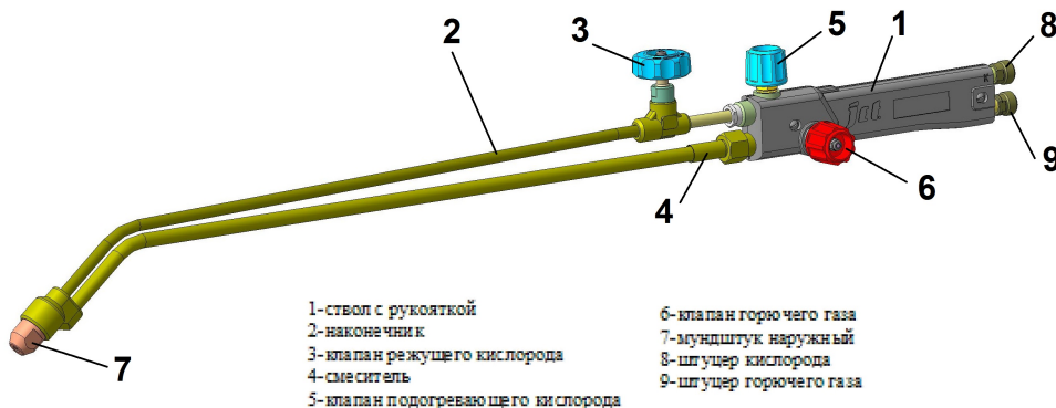
Рис. 1 Резак РЗПу (800) ДЖЕТ 505 10 в сборе.
